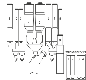
CAFFÈ IN GRANI x2 TRAMOGGE (configurazione valida per versione con gruppo espresso tradizionale + versione con gruppo caffè a camera variabile)
